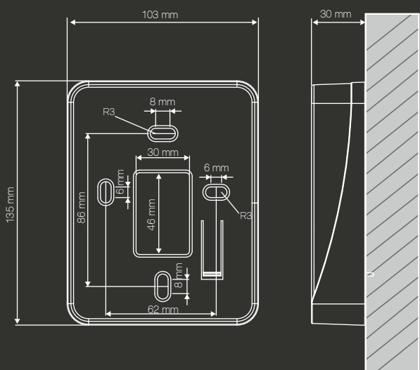
• 明裝孔位(正視圖)
